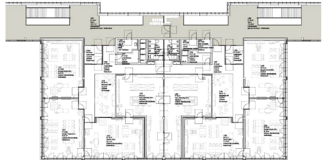
LPH3 Entwurf - Cluster NW Lernhaus 2 (Mitte)
