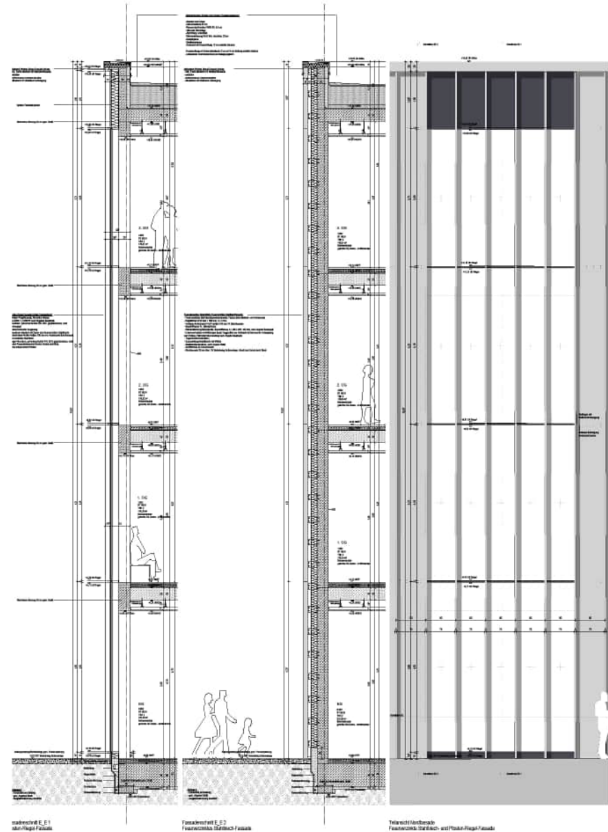
Nordfassade - Treppenriegel
