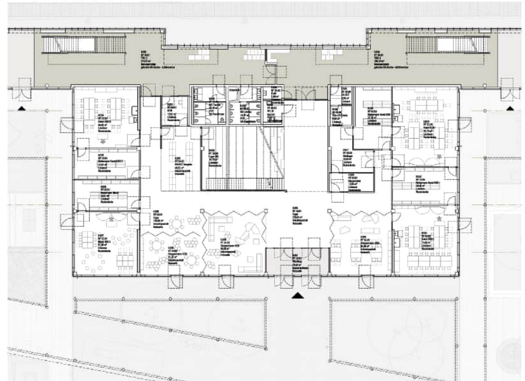
LPH3 Entwurf - Eingang / Halle / Sitztreppe Lernhaus 2 (Mitte)
